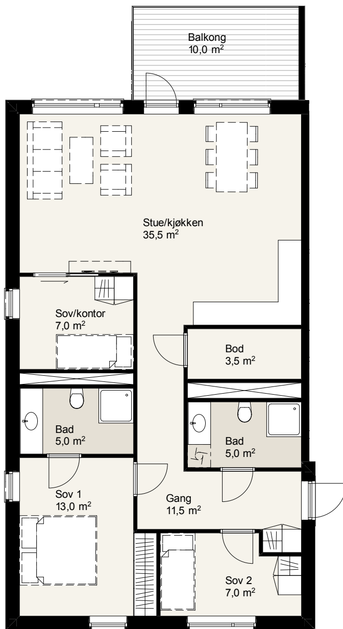
Leilighet A-201 94,5 m 2
